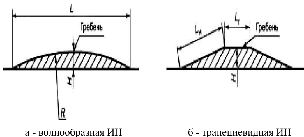
Рисунок 1 - Поперечные профили ИН
